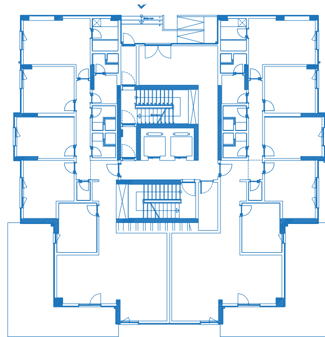
مخطط الدور الأرضي
