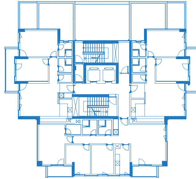
مخطط الأدوار (4-11)
